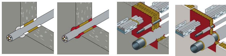
Eksempel på tætning af fuger ved installations-gennemføring i små huller med brandmastik
